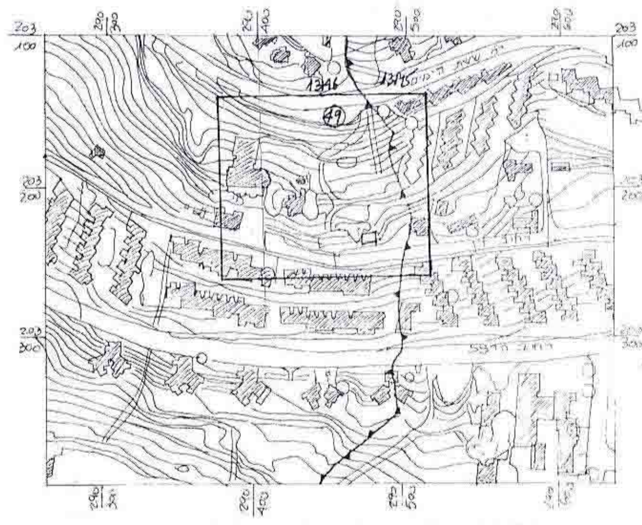
תוכנית סביבה - ק.כ. 1:2500
