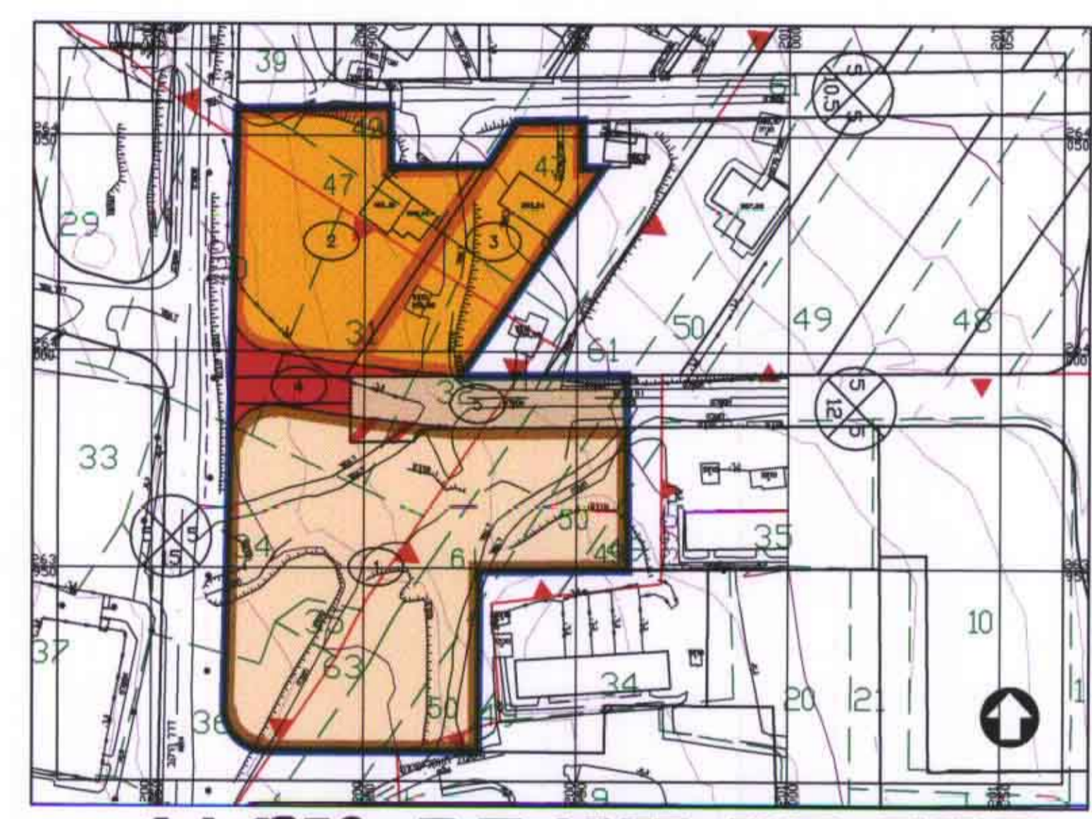
תכנית מצב מוצע ק.ת. 1250 : 1
