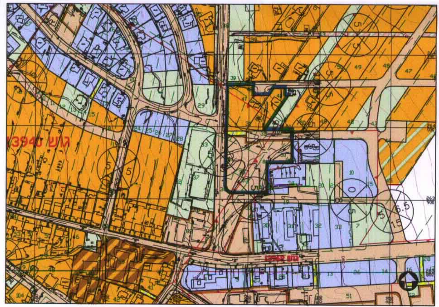
קטע מתכנית ראש פינה 5626 ק.ת. 2500 : 1
