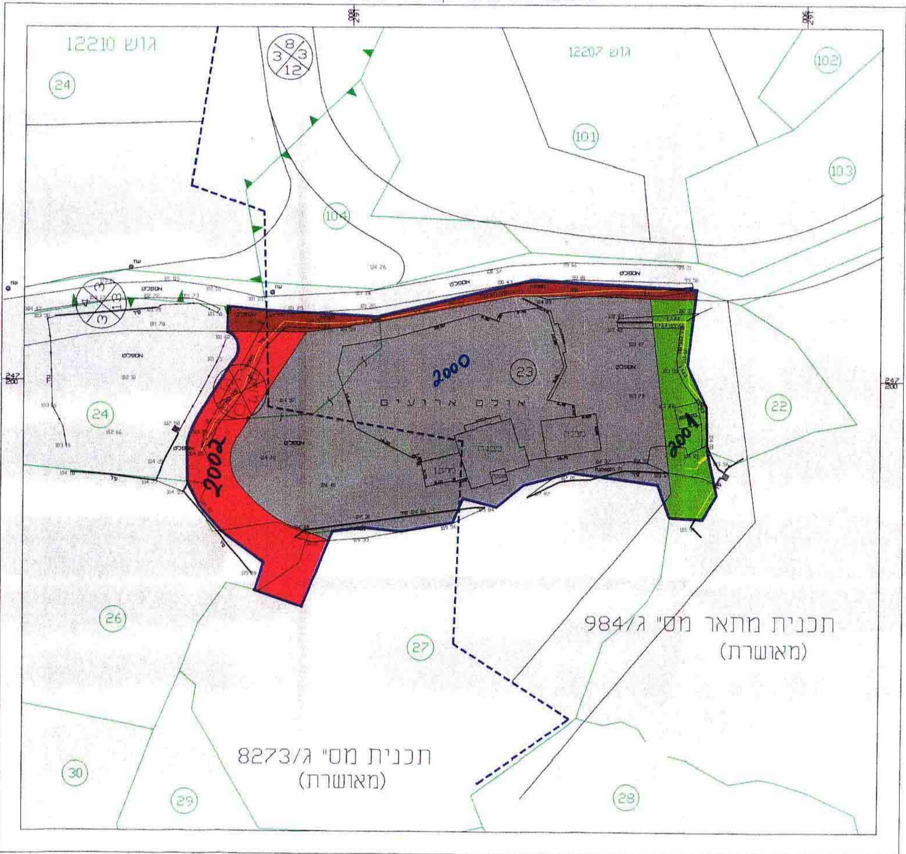
מצב מוצע קנ"מ 1:500
