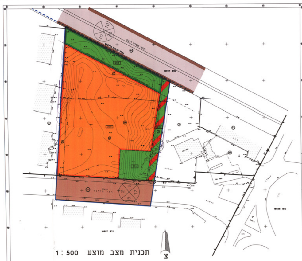
תכנית מצב קיים 1:500
