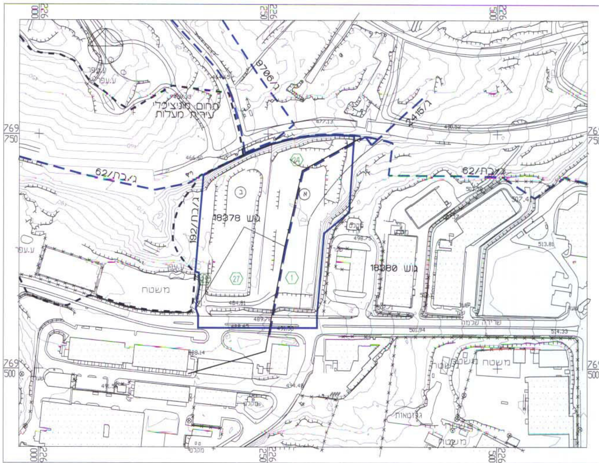
תכנית סביבה 1:2500
