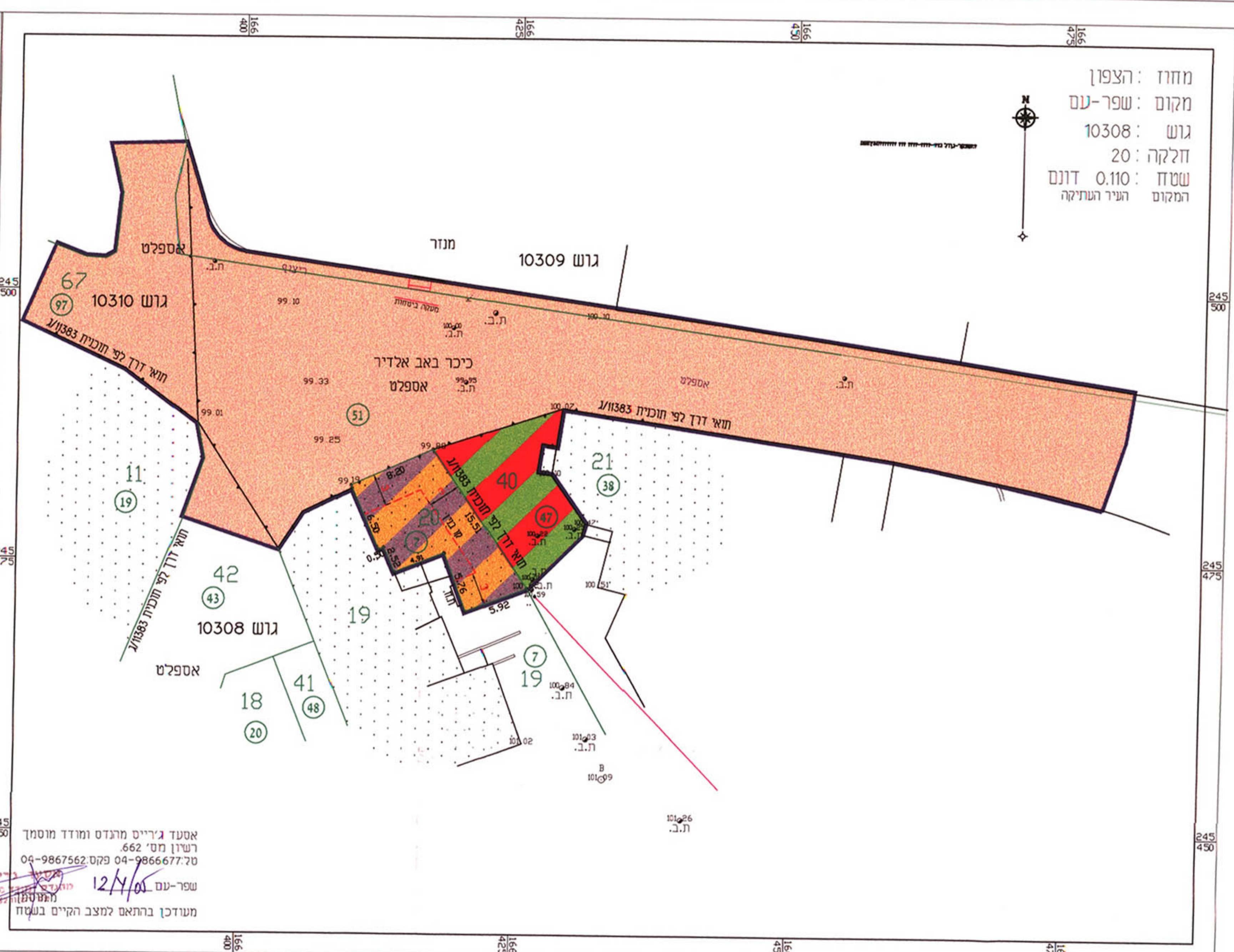
תכנית מצב קיים קני"מ 1:250
