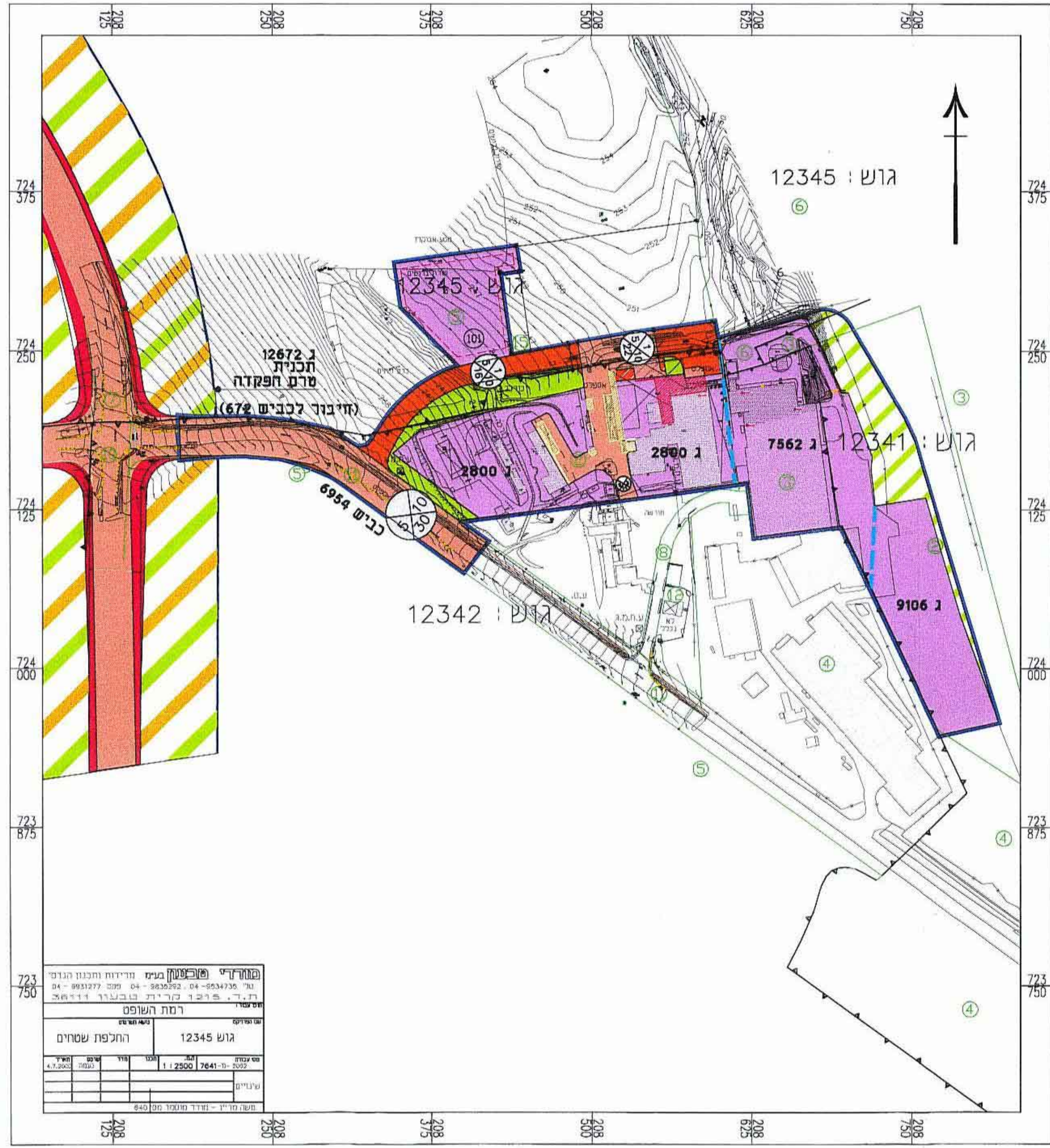
מצב מוצע 1:2500
