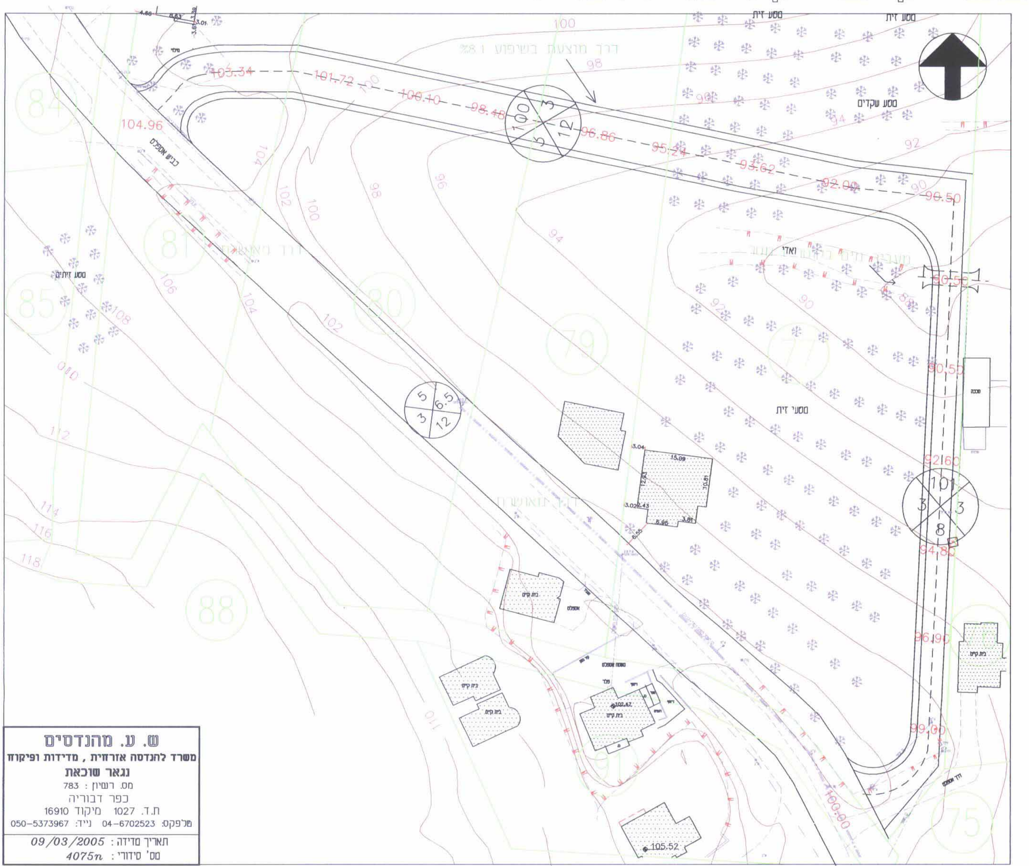
תכנית הדרך המוצעת ק.מ. 1:500
