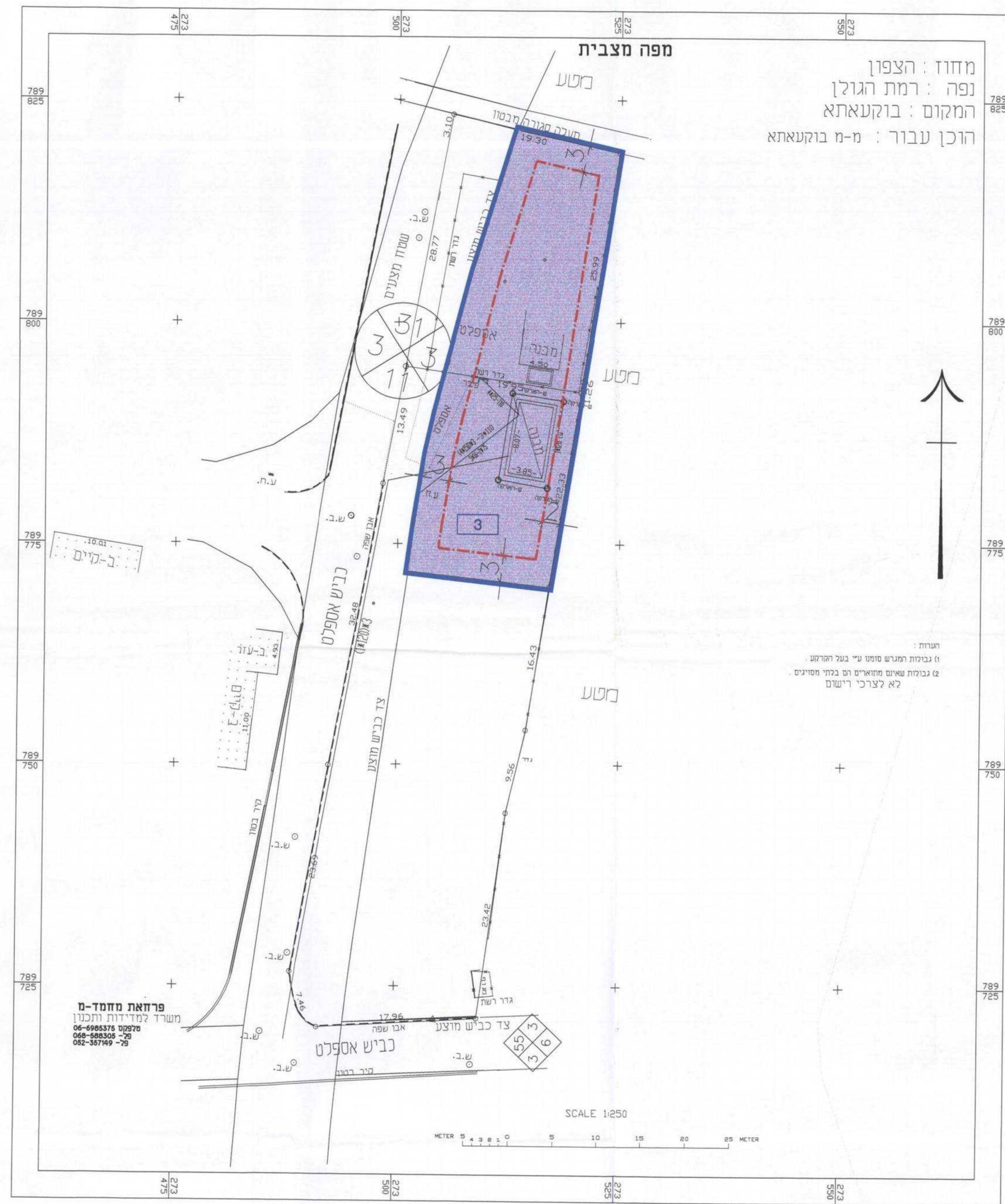
3 מתקנים הנדסיים מצב מוצע 1:250
