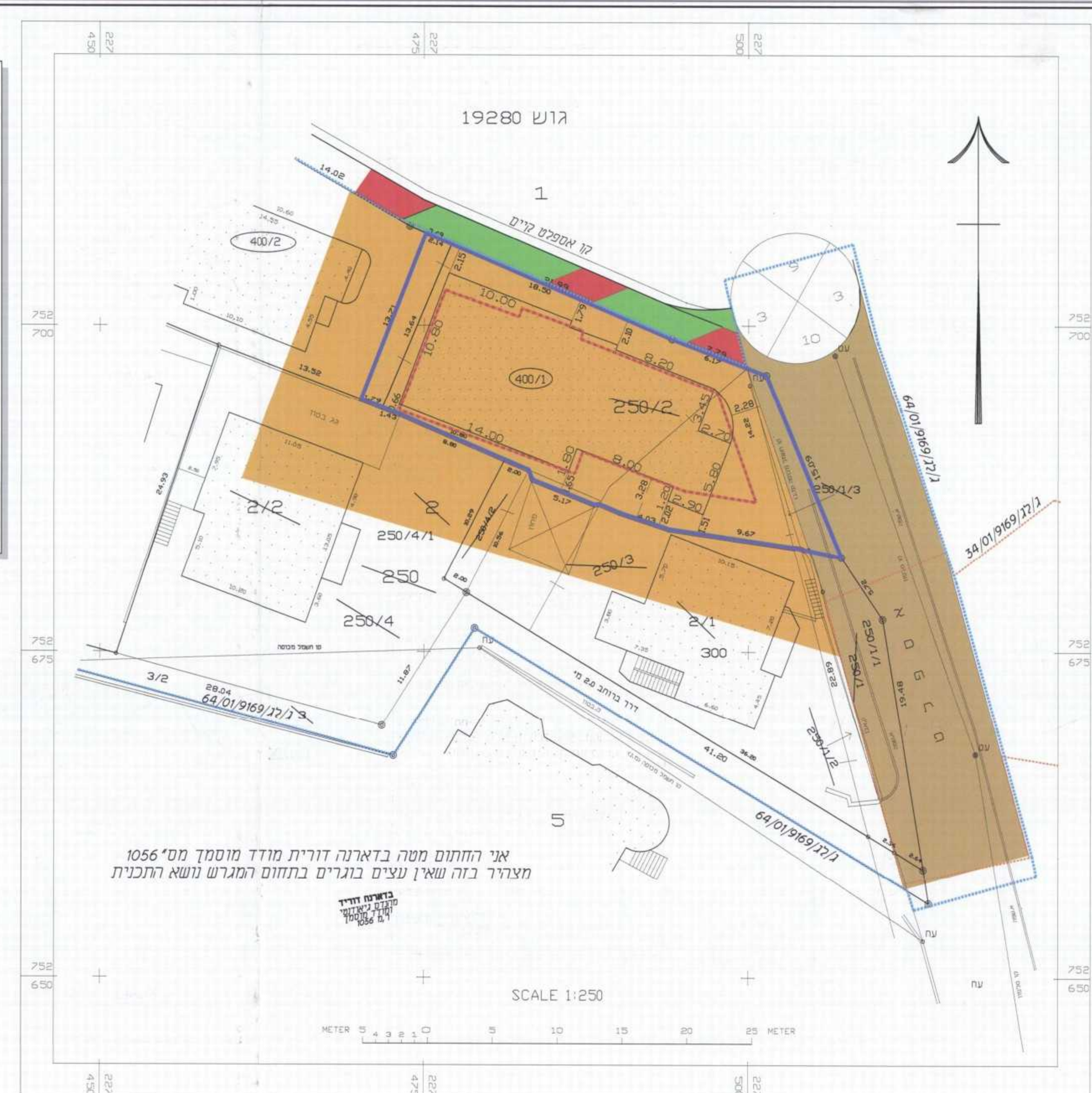
מצב מאושר קני"מ 1:250
