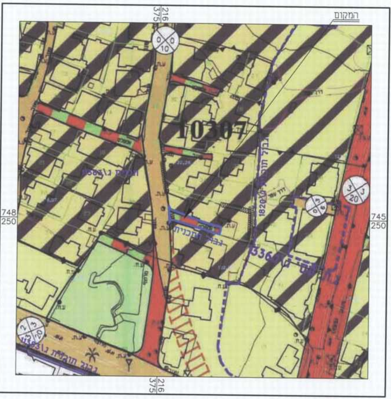
תרשים סביבה לפי ג/11383 קני"מ 1 : 1,250
