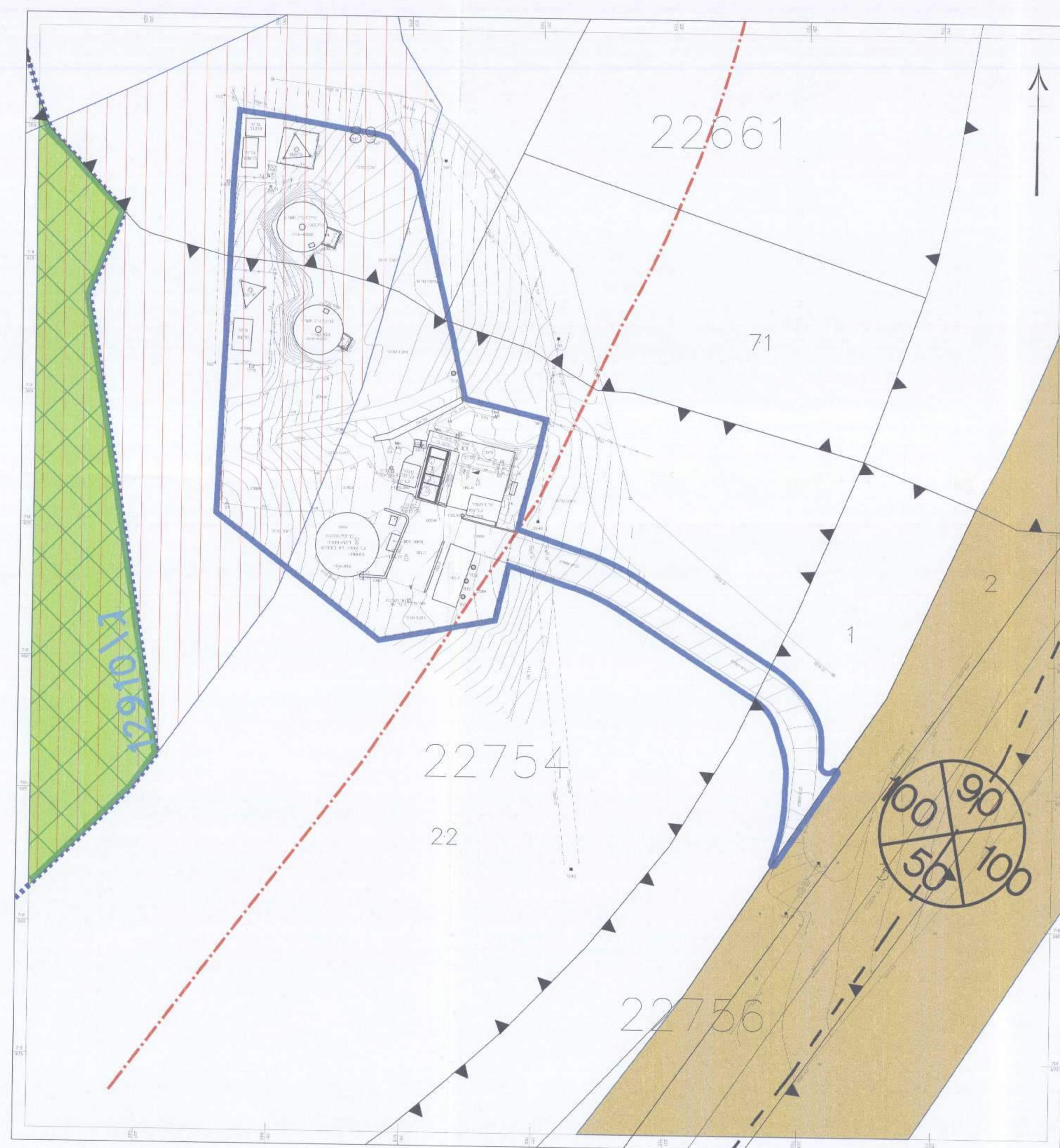
מצב מאושר קנ"מ 1 : 500
