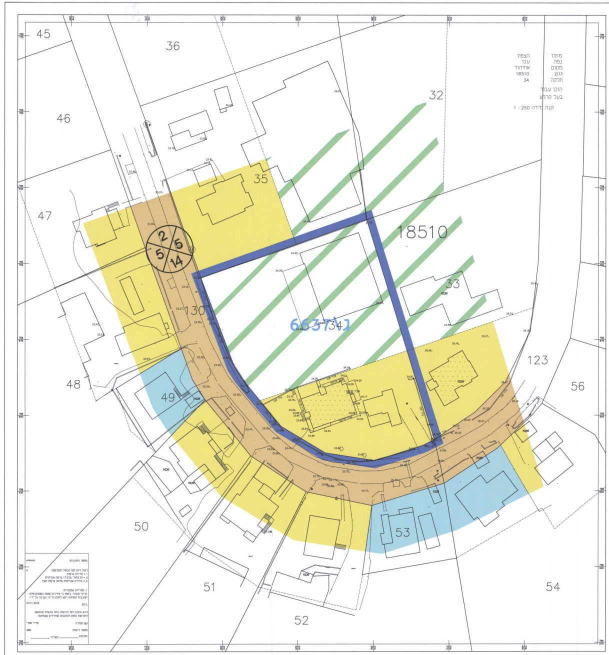
מצב מאושר 1:500
