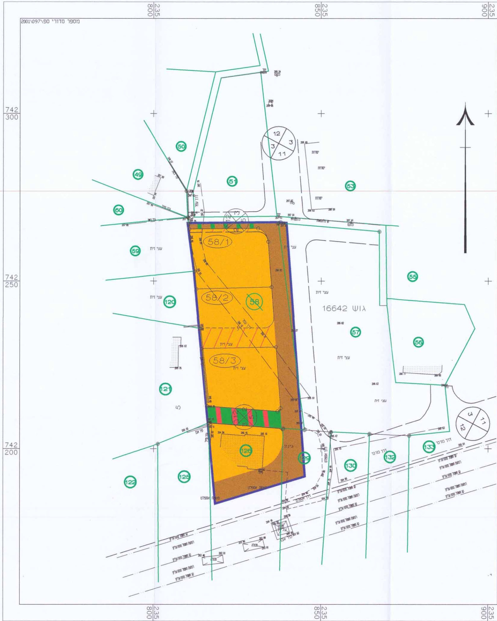
תכנית מצב מוצע קנ"מ 1:500
