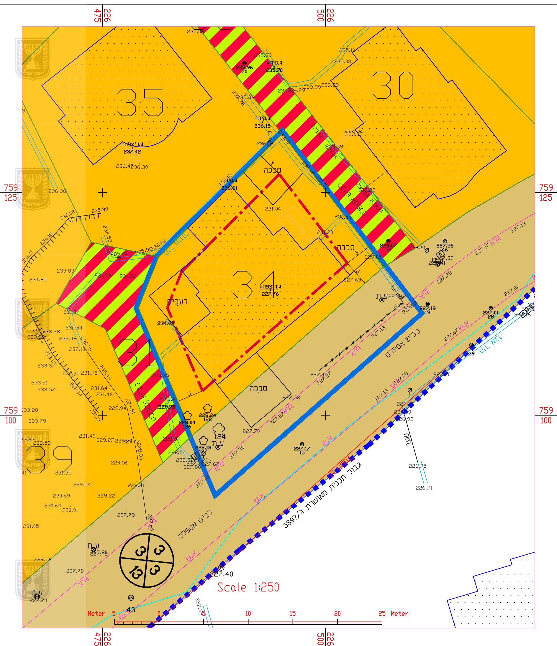
תרשים סביבה לפי תכנית מאושרת ג/3897 קנ"מ 1:250
