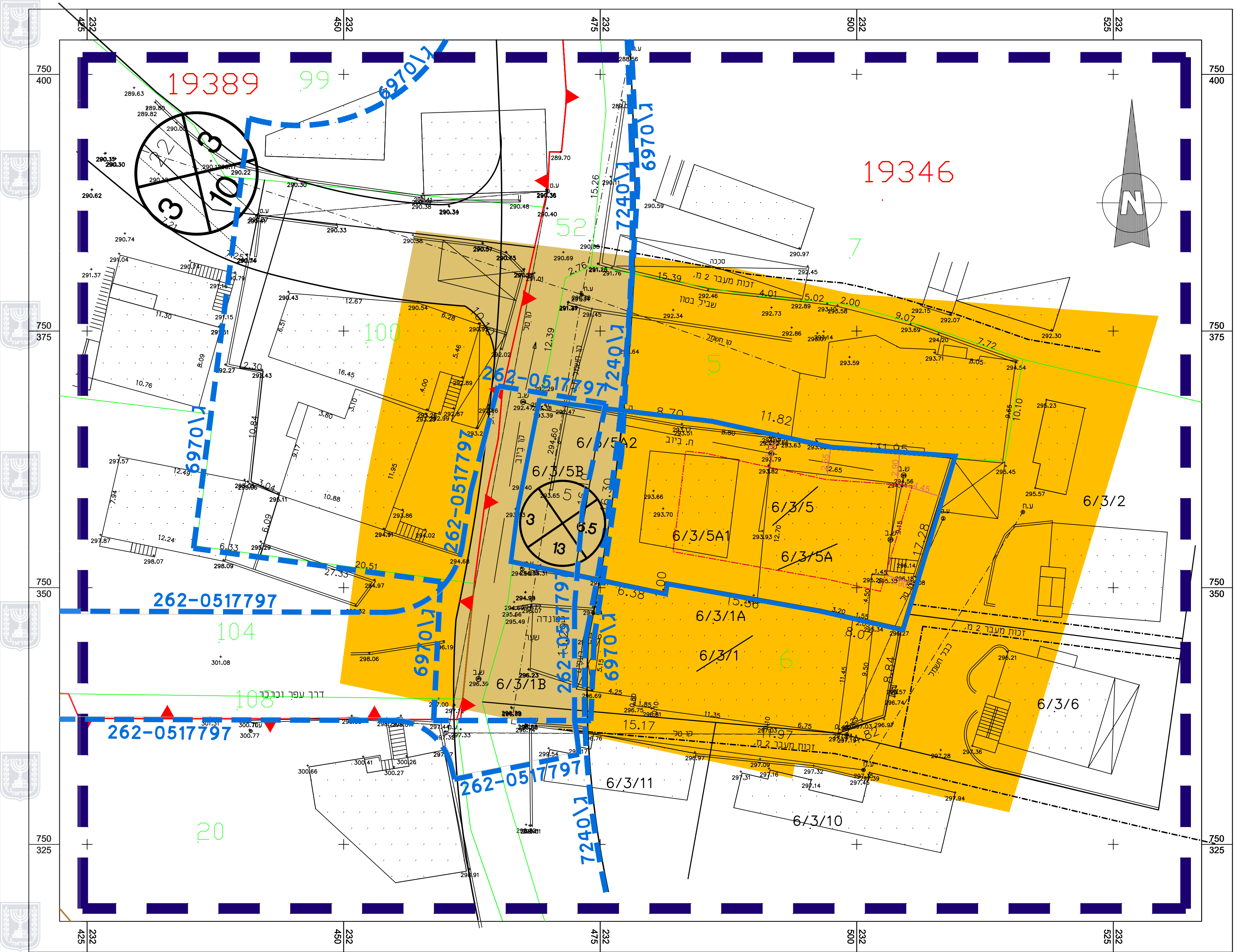
מצב קיים : קנ"מ 1:250
