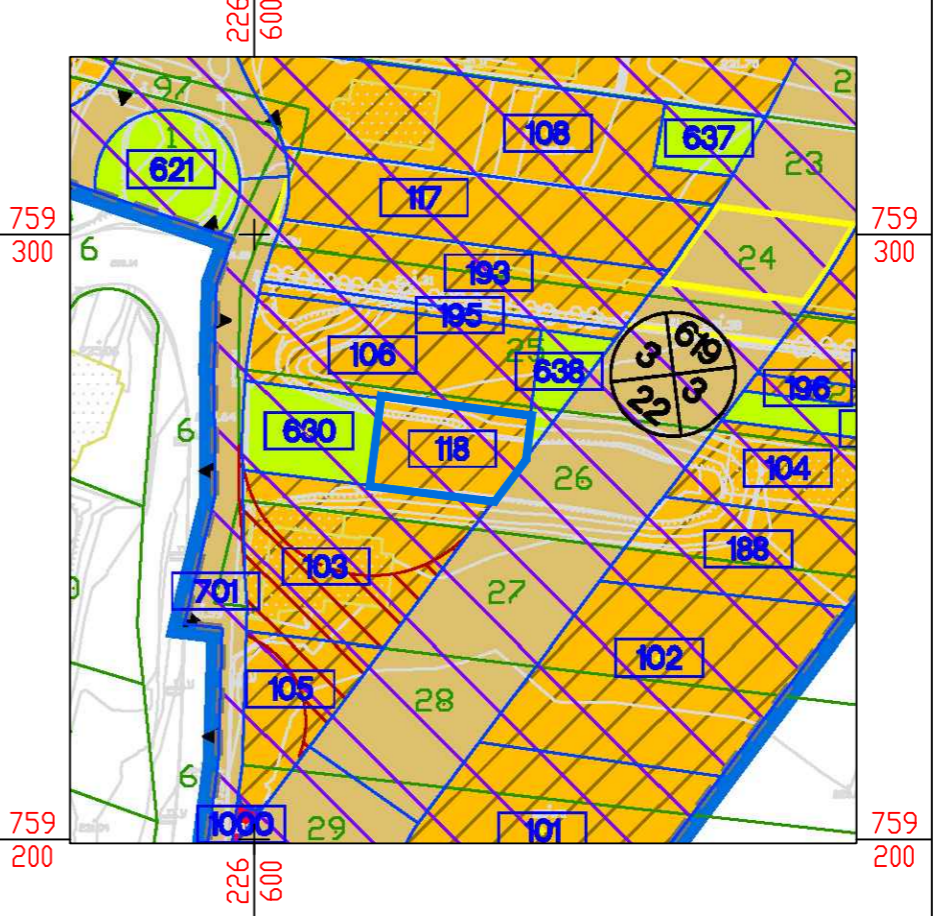
תרשים סביבה קני"מ 1:1250 לפי תוכנית מאושרת בכ/מק/15421/5/14
