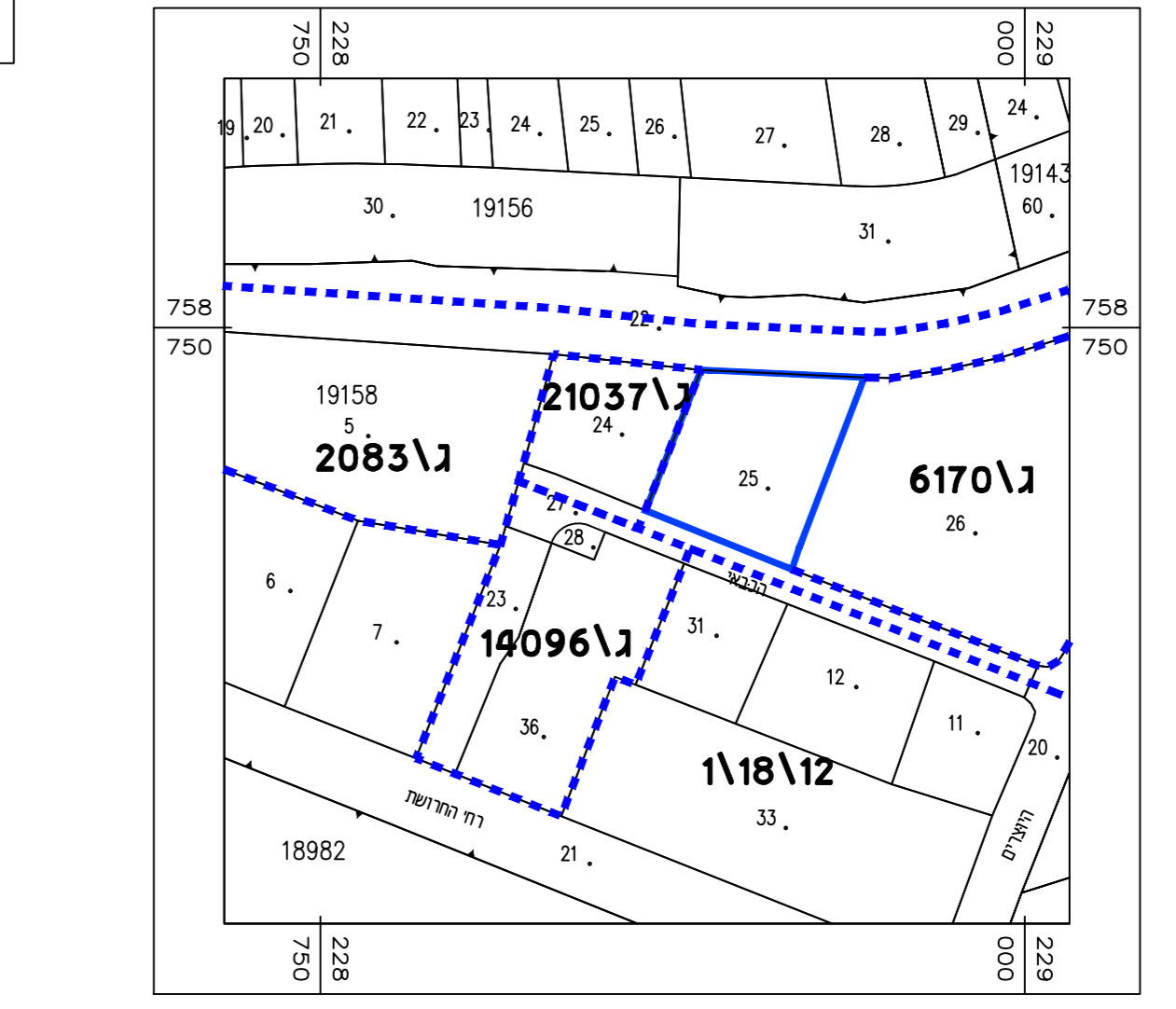
תרשים סביבה קנה מידה 1:2500
